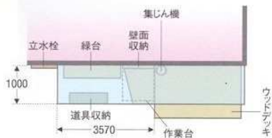
古河さんの工房上面図 *単位はmm
